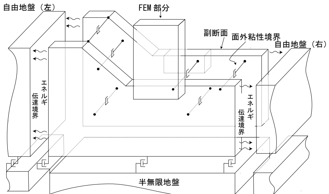
b. 両外方向の地盤を副断面とする場合
